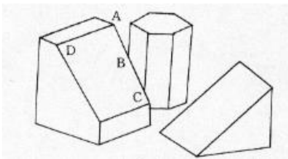
积木世界
